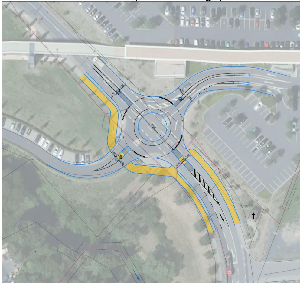
Abbildung 2: skizzenhafter Entwurf Kreisverkehr an K5
