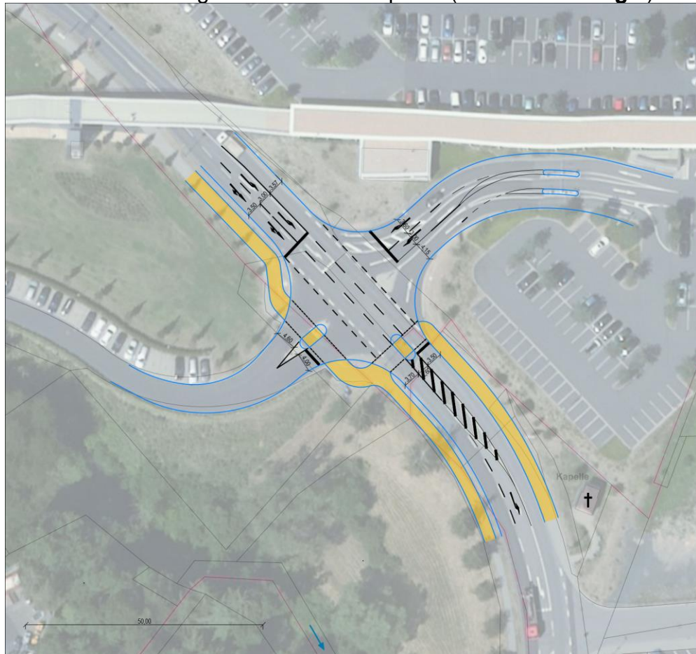
Abbildung 3: skizzenhafter Entwurf Lichtsignalanlage an K5
